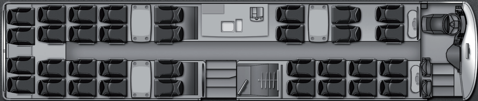
Floorplan Mercedes-Benz Travego S34/1 (34 Sitzplätze - davon 12 Plätze an Tischen)
